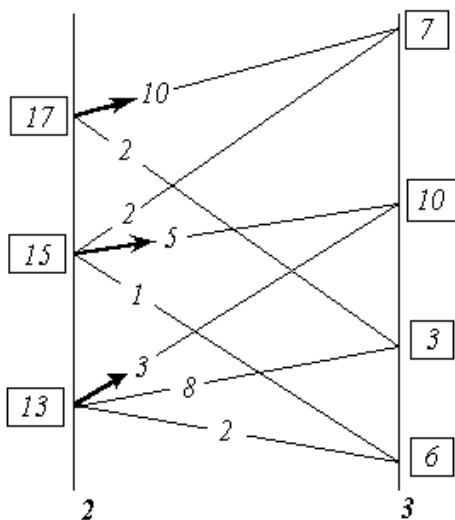
Рис. 9. К СУЩЕСТВУ МЕТОДА ДИНАМИЧЕСКОГО ПРОГРАММИРОВАНИЯ. АНАЛИЗ ПЕРЕХОДОВ.
