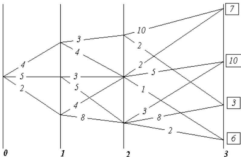
Рис. 8. К СУЩЕСТВУ МЕТОДА ДИНАМИЧЕСКОГО ПРОГРАММИРОВАНИЯ. МАТРИЦА ВОЗМОЖНОСТЕЙ.
