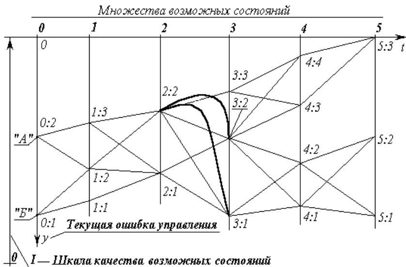
Рис. 11. ДИНАМИЧЕСКОЕ ПРОГРАММИРОВАНИЕ, РАЗЛИЧИЕ И ДОСТАТОЧНО ОБЩАЯ ТЕОРИЯ УПРАВЛЕНИЯ
