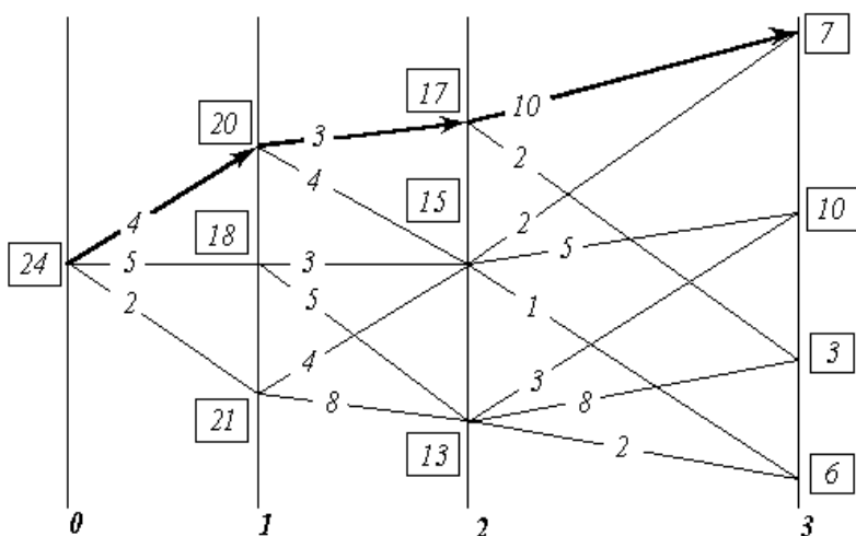
Рис. 10. К СУЩЕСТВУ МЕТОДА ДИНАМИЧЕСКОГО ПРОГРАММИРОВАНИЯ. ОПТИМАЛЬНАЯ ТРАЕКТОРИЯ.
