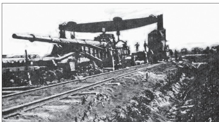
Монтаж «Колоссаль» на железнодорожную платформу
